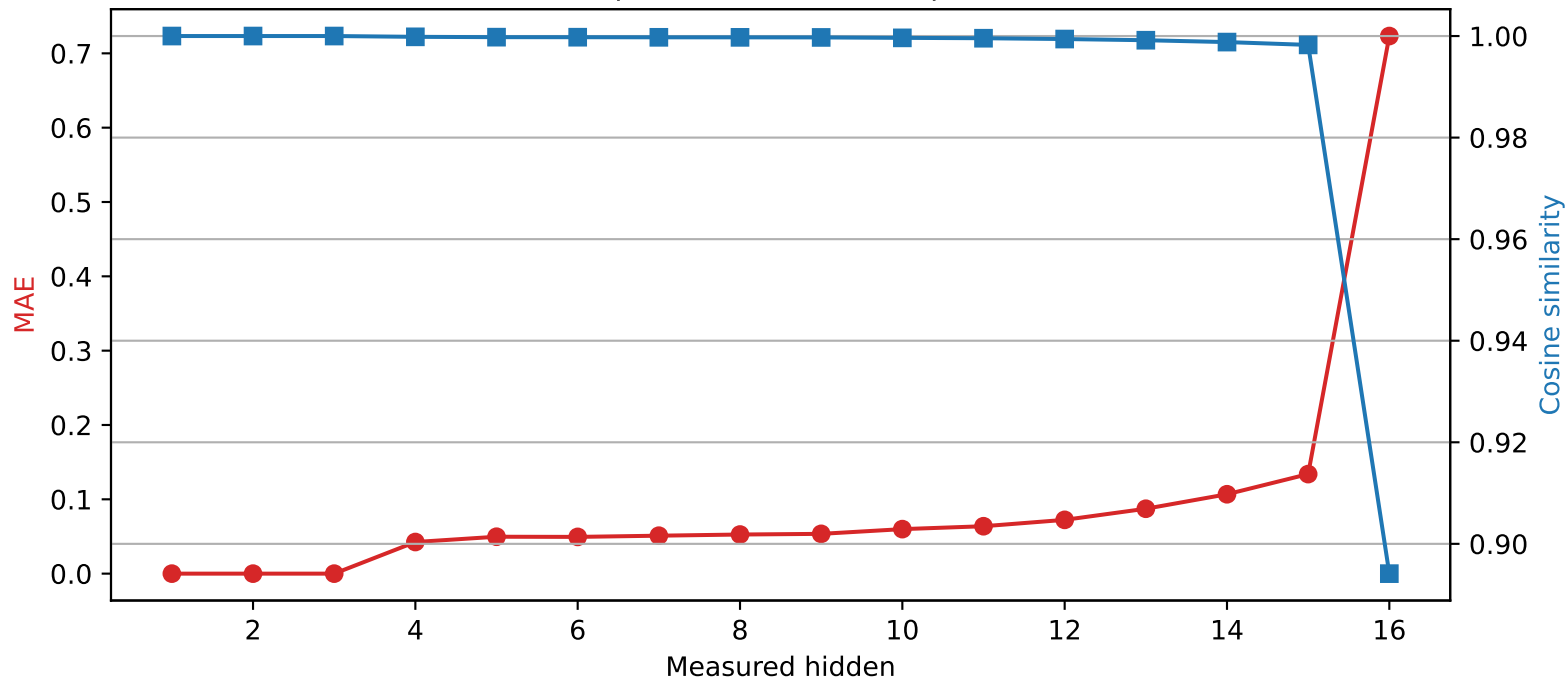
Llama-3.2-1B | Quantized layer 3 | float64 \rightarrow int2
