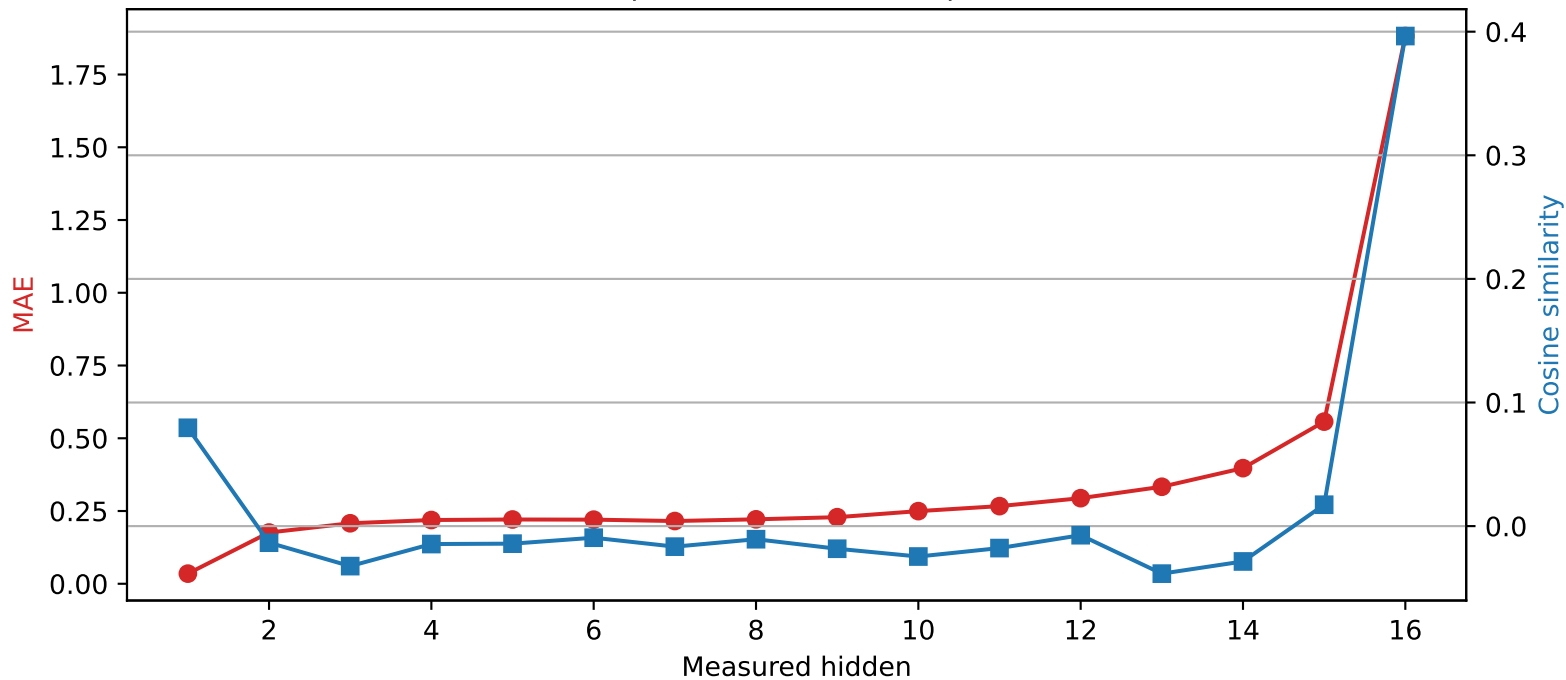
Llama-3.2-1B | Quantized layer 0 | float64 \rightarrow int2
