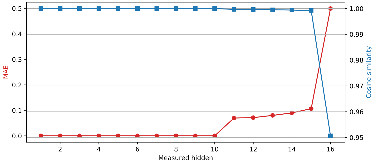
Llama-3.2-1B | Quantized layer 10 | float64 \rightarrow int2
