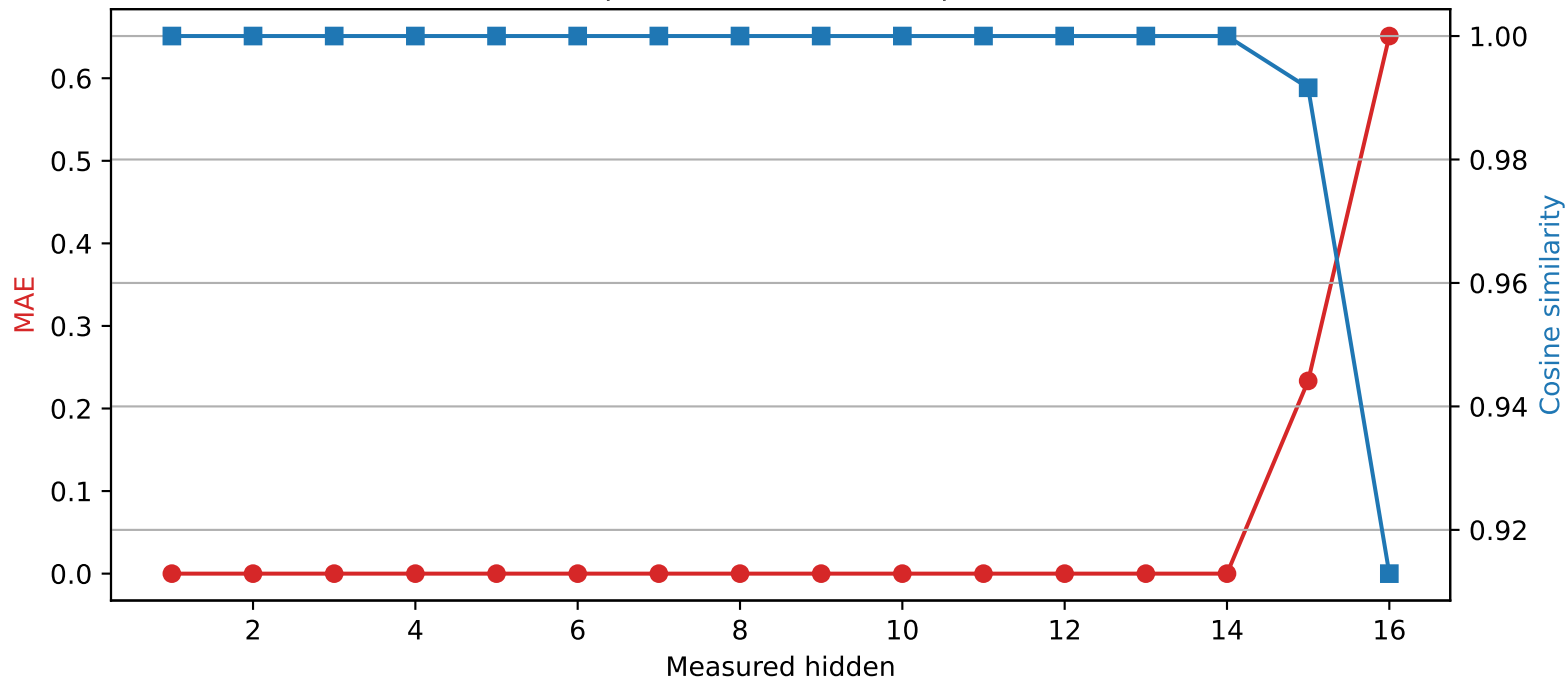
Llama-3.2-1B | Quantized layer 14 | float64 \rightarrow int2
