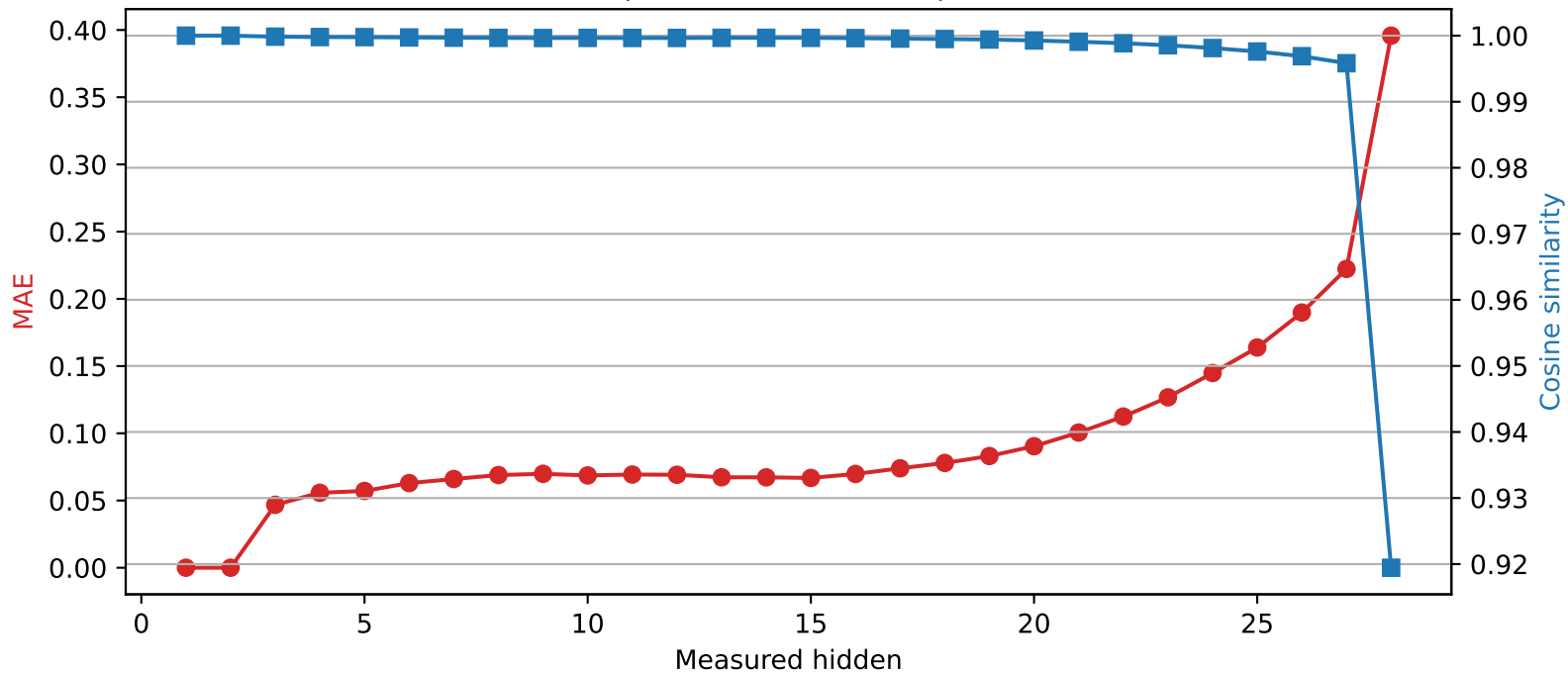
Llama-3.2-3B | Quantized layer 2 | float16 \rightarrow int4
