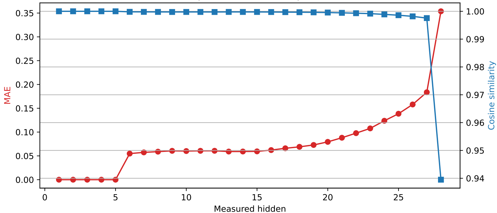
Llama-3.2-3B | Quantized layer 5 | float16 \rightarrow int4
