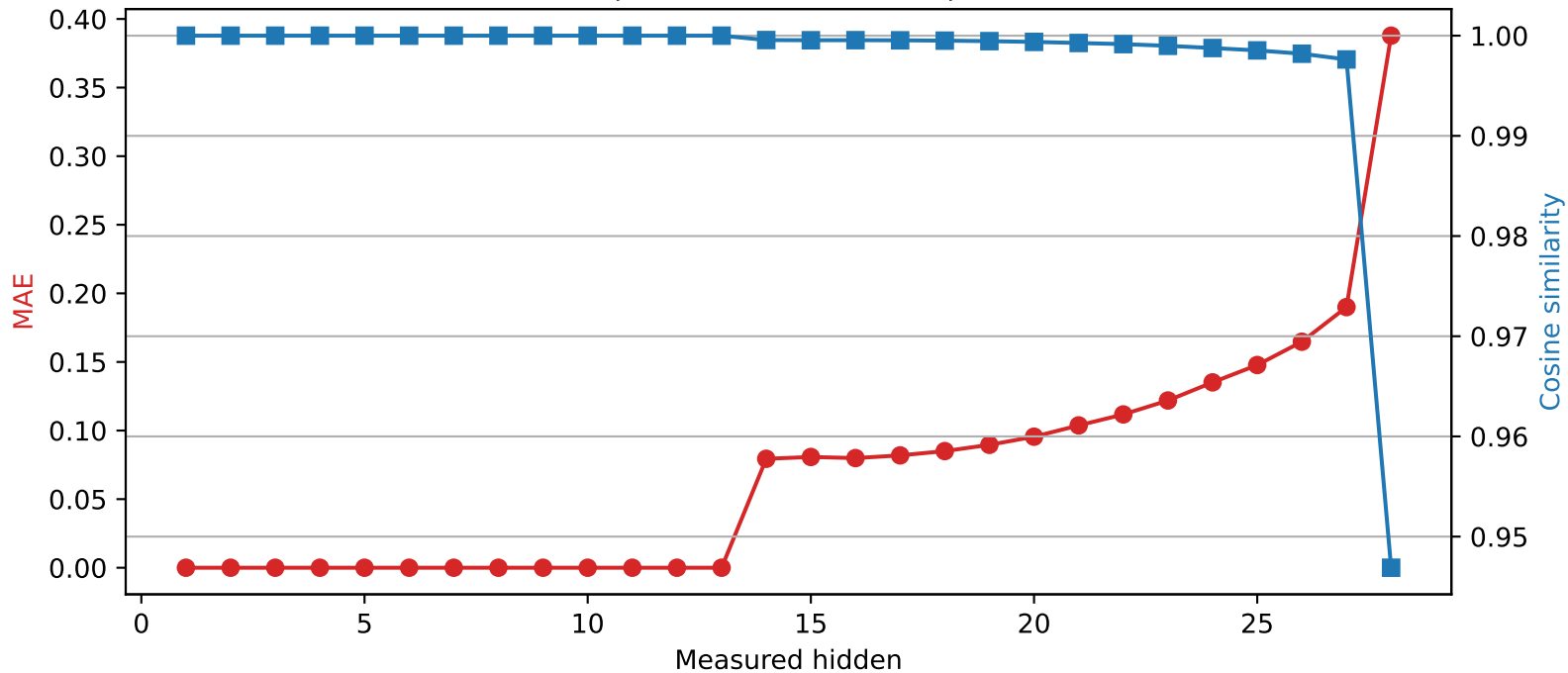
Llama-3.2-3B | Quantized layer 13 | float16 \rightarrow int4
