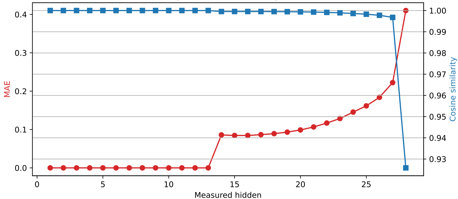
Llama-3.2-3B | Quantized layer 13 | float32 \rightarrow int4
