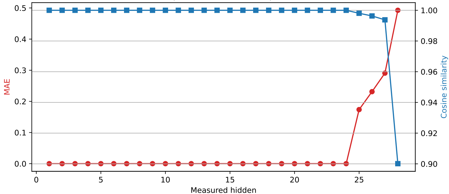
Llama-3.2-3B | Quantized layer 24 | float32 \rightarrow int4
