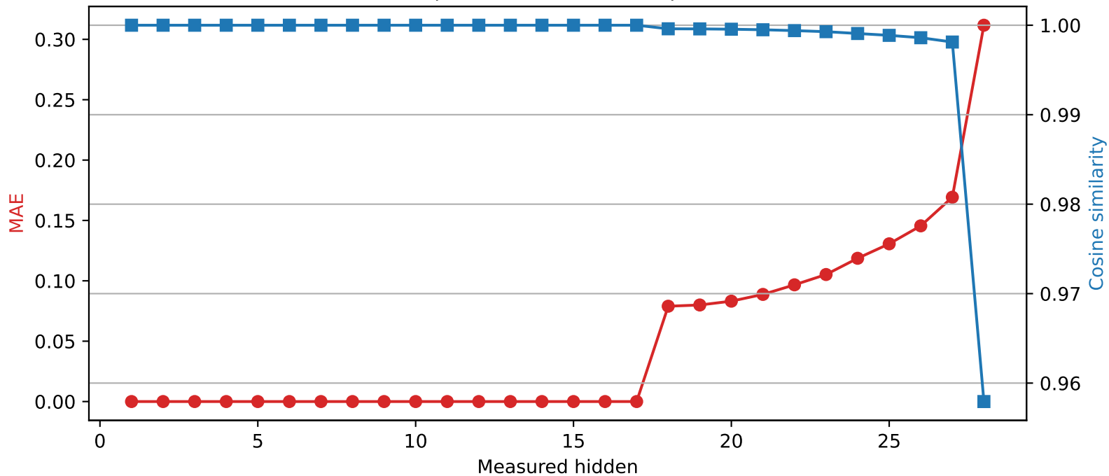
Llama-3.2-3B | Quantized layer 17 | float32 \rightarrow int4
