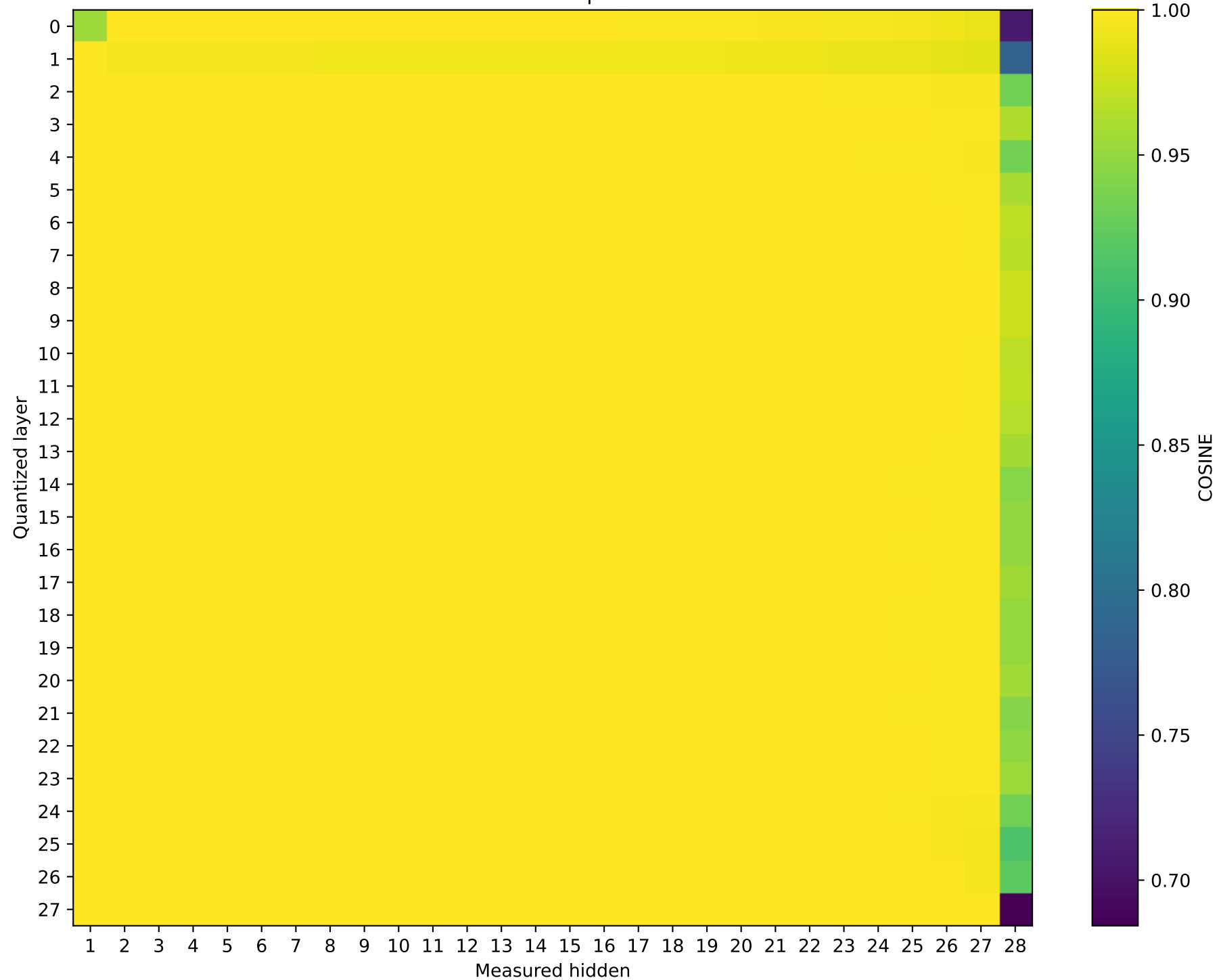
Model: Llama-3.2-3B | float64 → int4
