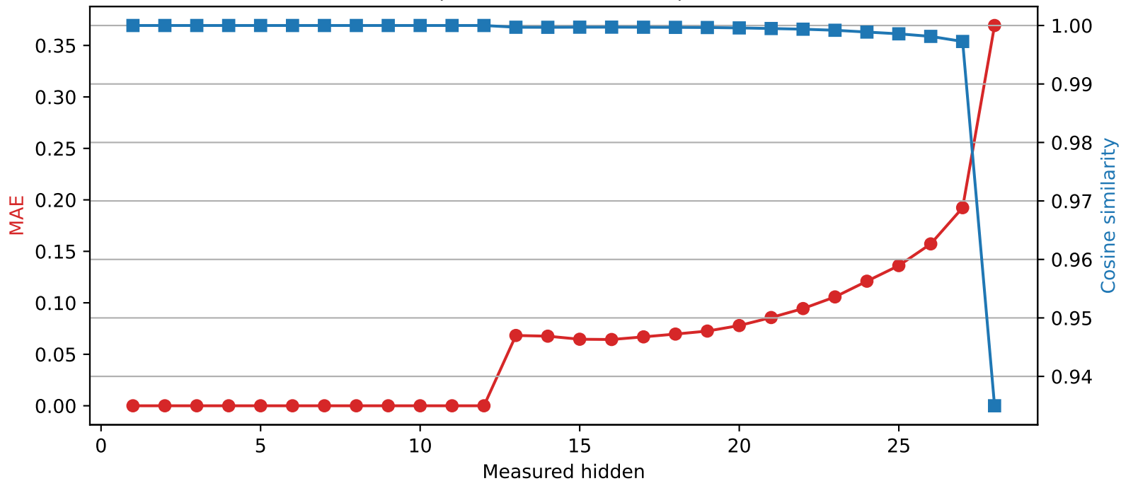
Llama-3.2-3B | Quantized layer 12 | float64 \rightarrow int4
