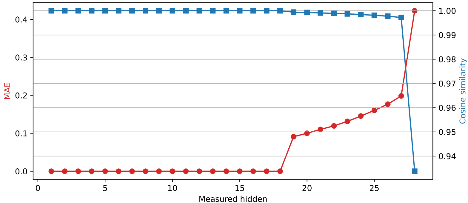
Llama-3.2-3B | Quantized layer 18 | float64 \rightarrow int4
