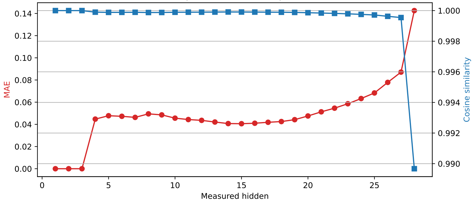
Llama-3.2-3B | Quantized layer 3 | float64 \rightarrow int4
