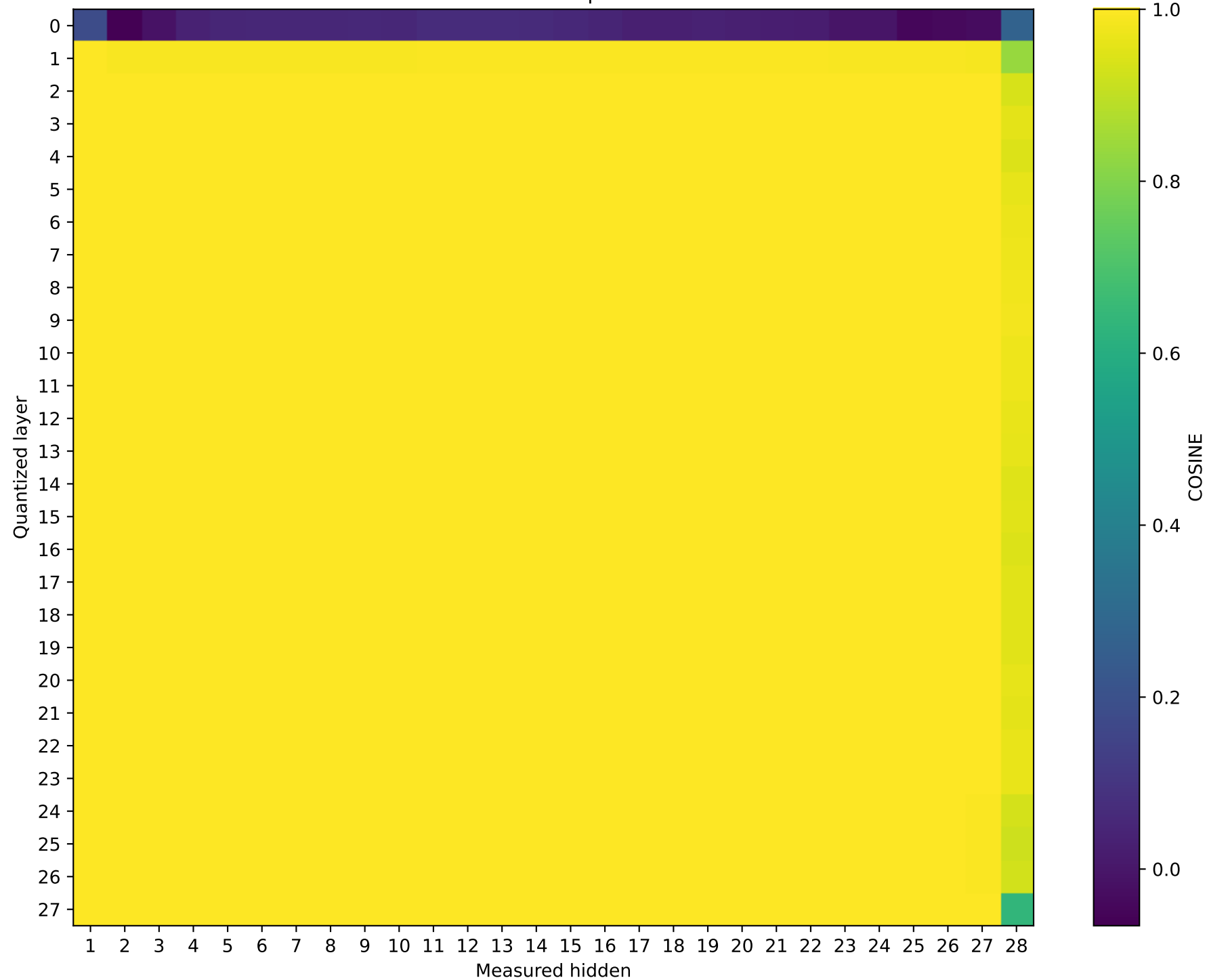
Model: Llama-3.2-3B | float16 → int2
