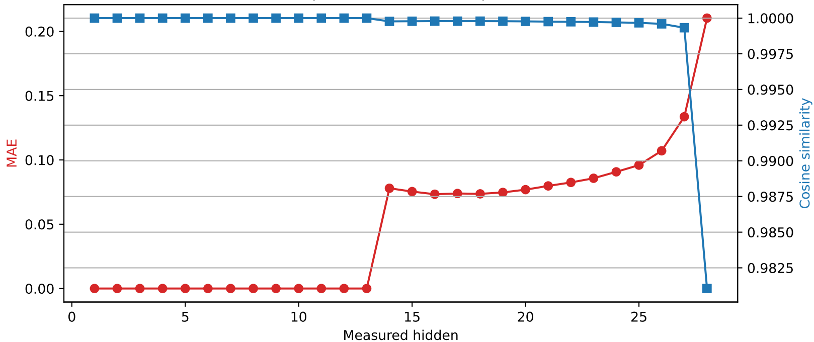
Llama-3.2-3B | Quantized layer 13 | float16 \rightarrow int2
