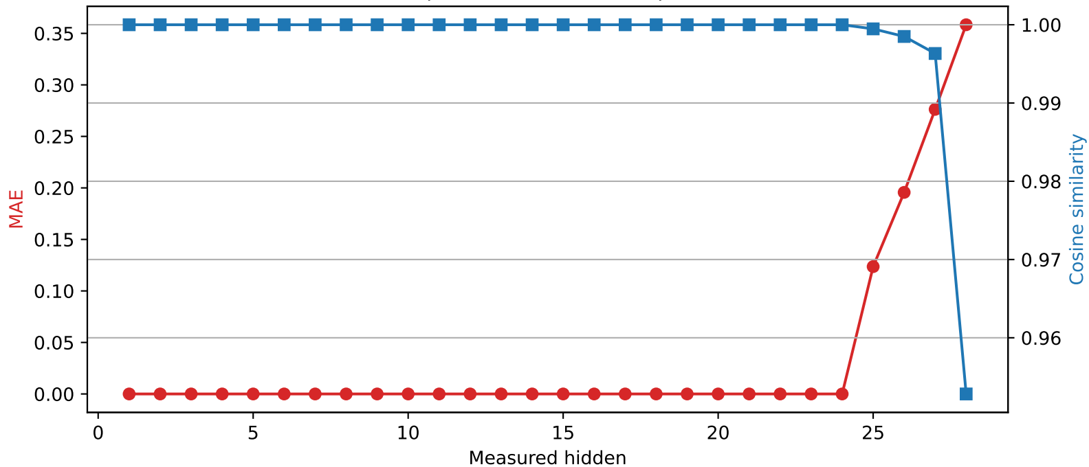
Llama-3.2-3B | Quantized layer 24 | float16 \rightarrow int2
