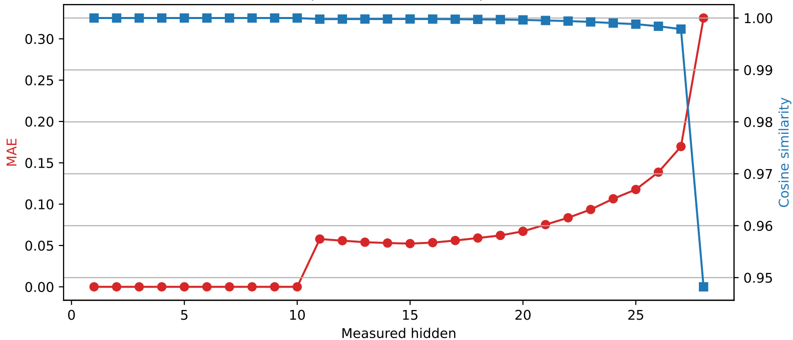
Llama-3.2-3B | Quantized layer 10 | float16 \rightarrow int2
