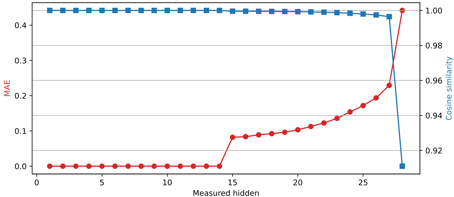
Llama-3.2-3B | Quantized layer 14 | float16 \rightarrow int2
