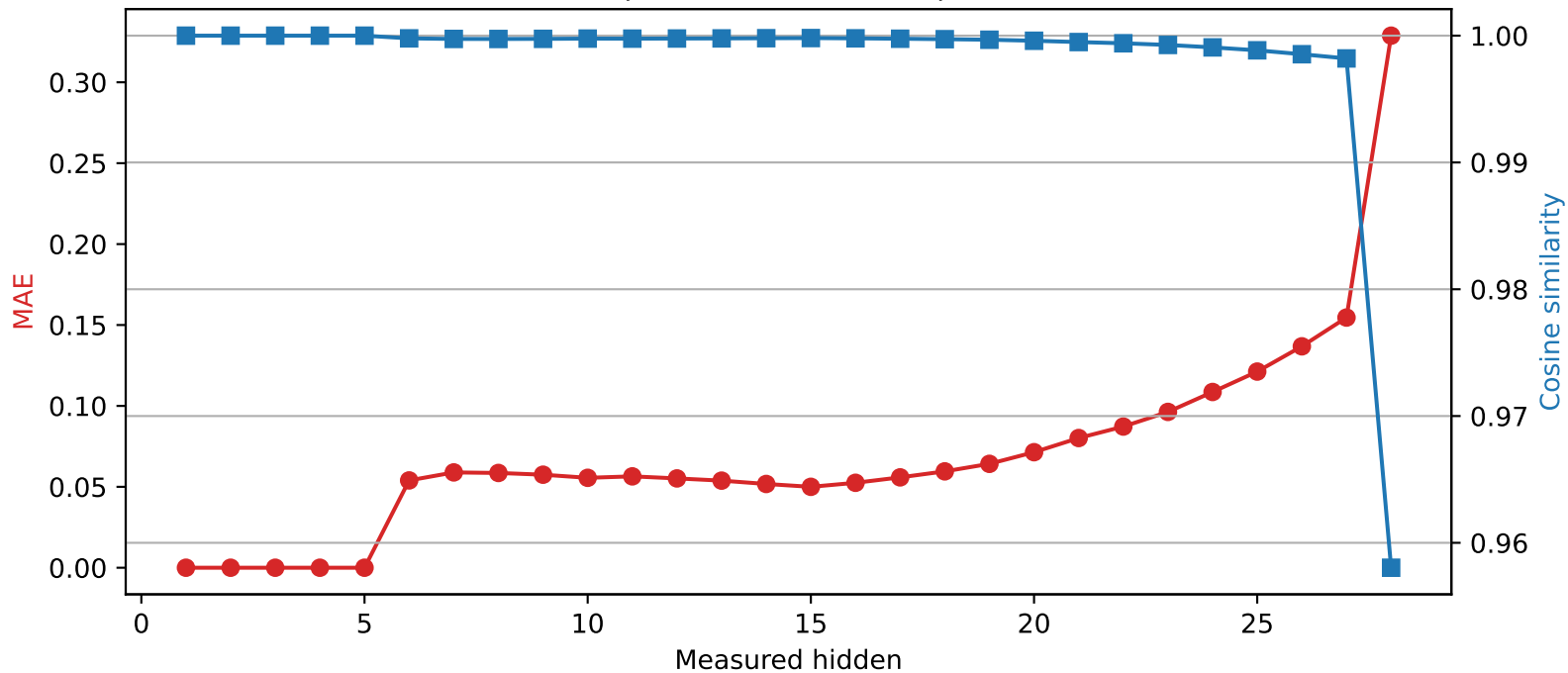
Llama-3.2-3B | Quantized layer 5 | float16 \rightarrow int2
