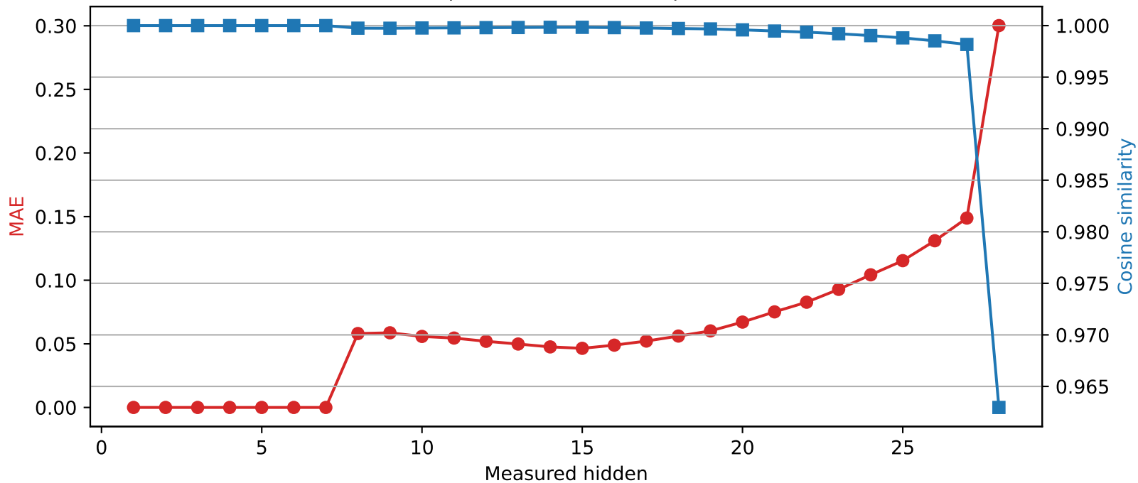
Llama-3.2-3B | Quantized layer 7 | float16 \rightarrow int2
