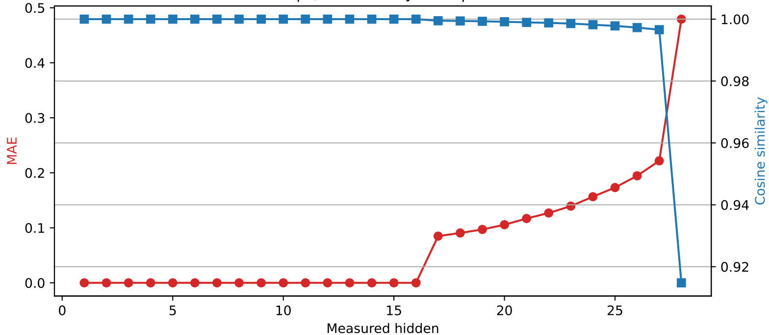
Llama-3.2-3B | Quantized layer 16 | float16 \rightarrow int2
