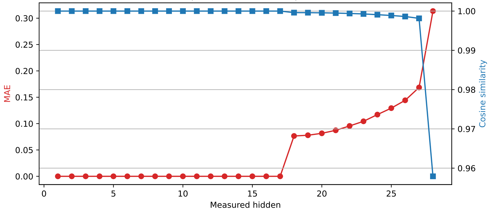
Llama-3.2-3B | Quantized layer 17 | float16 \rightarrow int2
