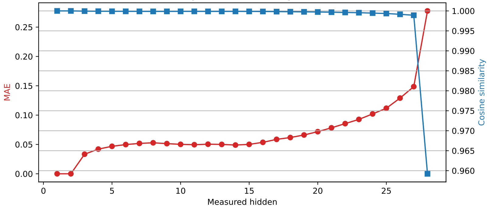
Llama-3.2-3B | Quantized layer 2 | float32 \rightarrow int2
