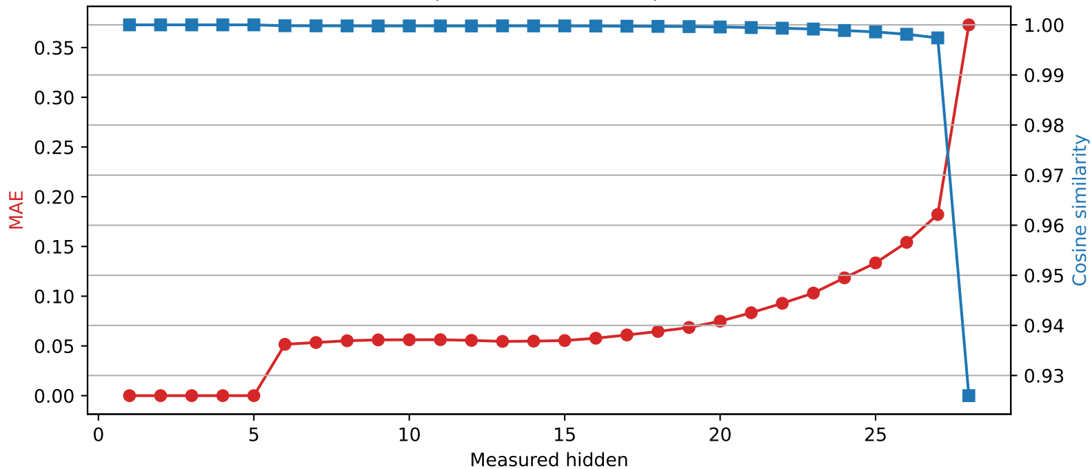
Llama-3.2-3B | Quantized layer 5 | float32 \rightarrow int2
