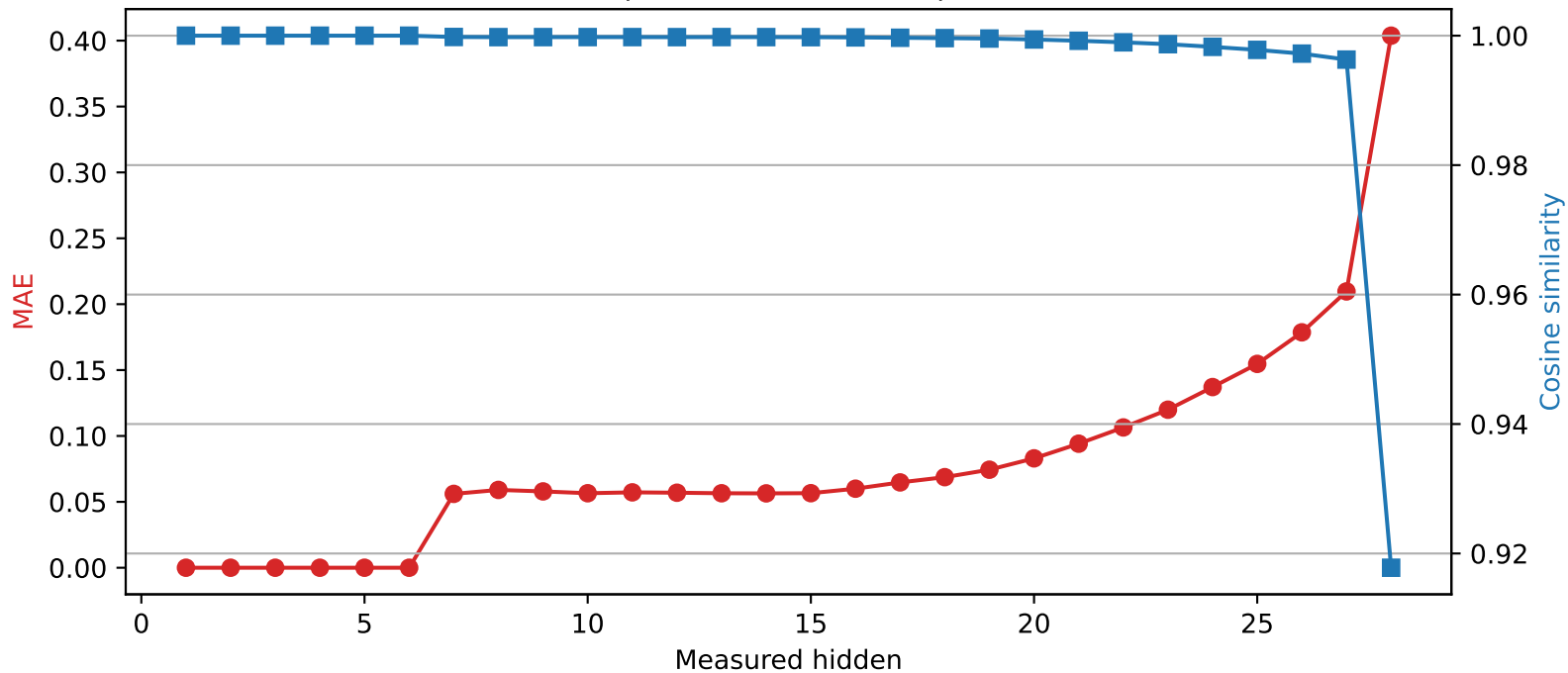
Llama-3.2-3B | Quantized layer 6 | float32 \rightarrow int2
