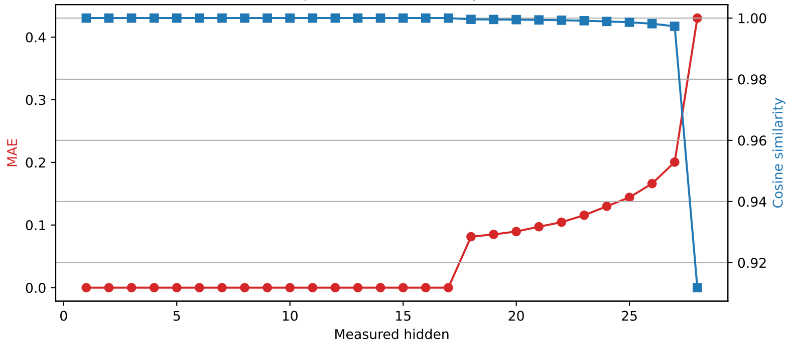
Llama-3.2-3B | Quantized layer 17 | float32 \rightarrow int2
