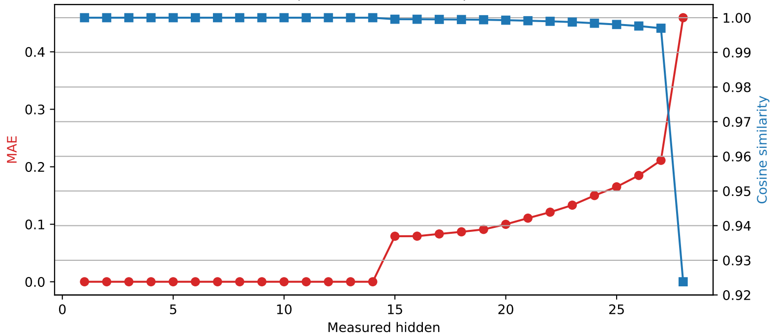
Llama-3.2-3B | Quantized layer 14 | float32 \rightarrow int2
