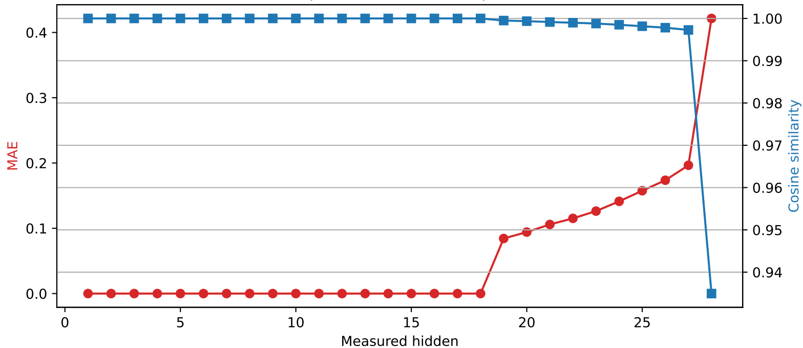
Llama-3.2-3B | Quantized layer 18 | float32 \rightarrow int2
