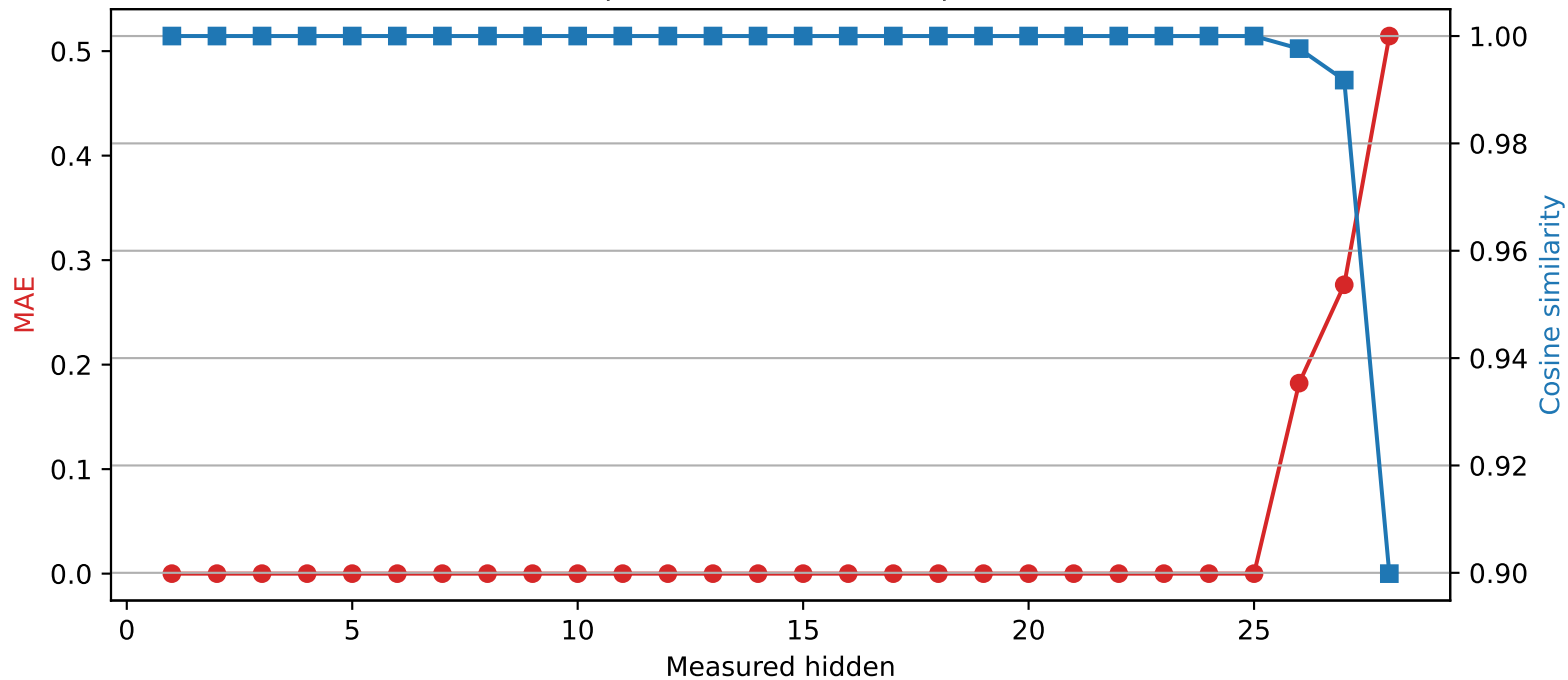
Llama-3.2-3B | Quantized layer 25 | float32 \rightarrow int2
