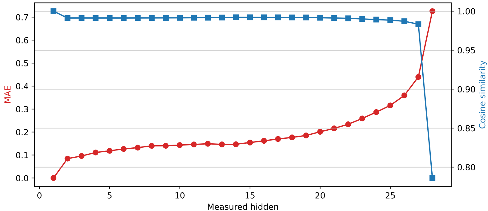
Llama-3.2-3B | Quantized layer 1 | float32 \rightarrow int2
