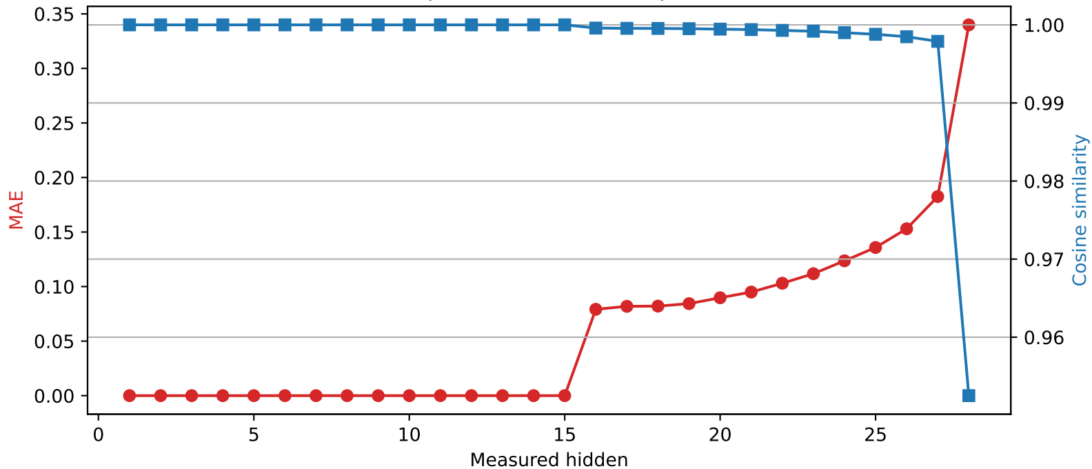
Llama-3.2-3B | Quantized layer 15 | float32 \rightarrow int2
