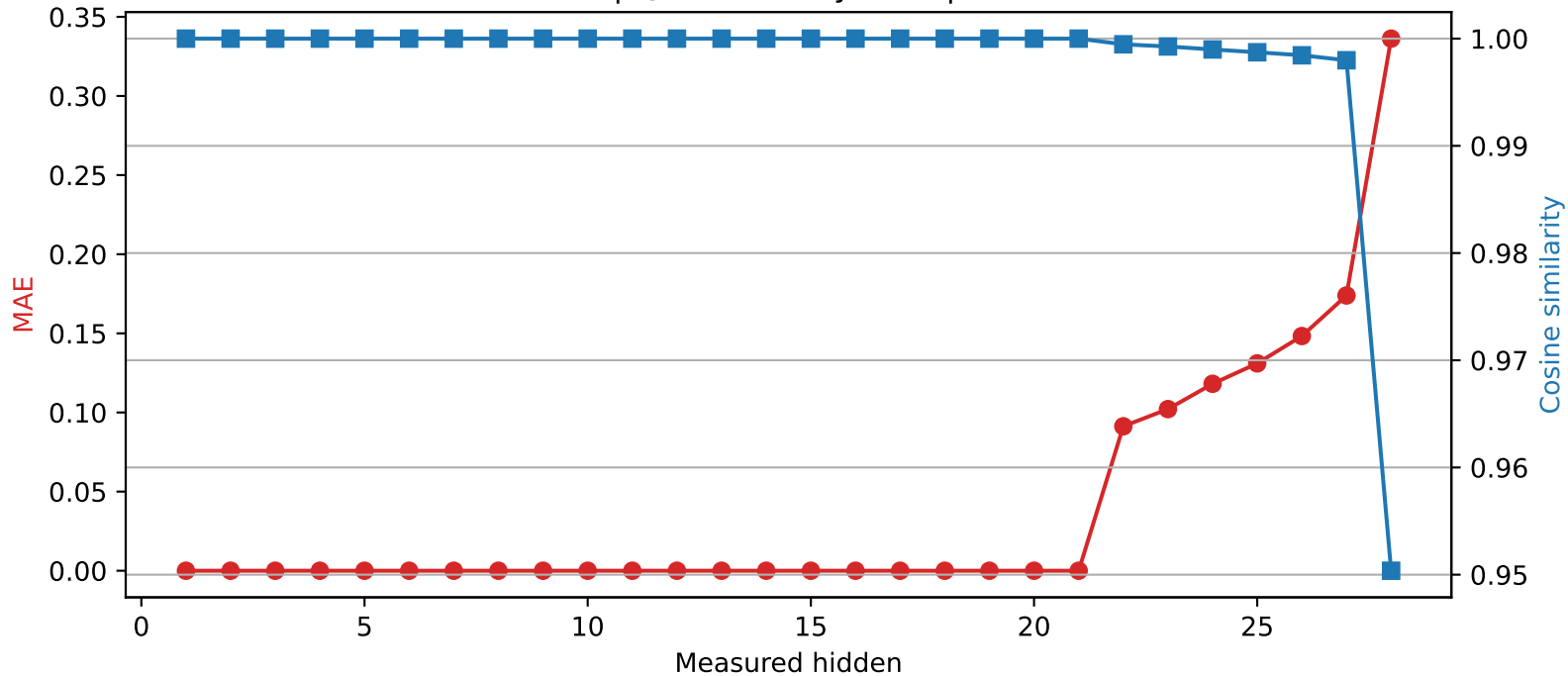
Llama-3.2-3B | Quantized layer 21 | float32 \rightarrow int2
