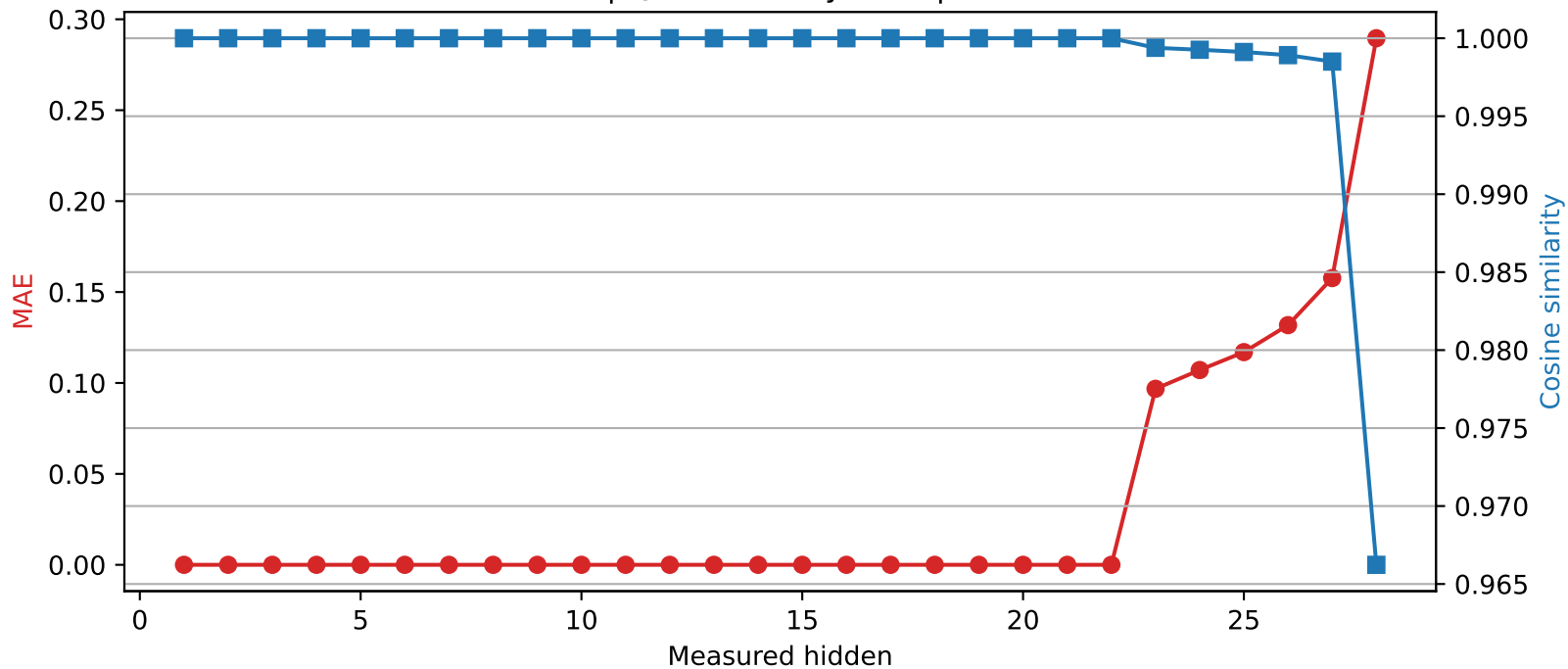
Llama-3.2-3B | Quantized layer 22 | float32 \rightarrow int2
