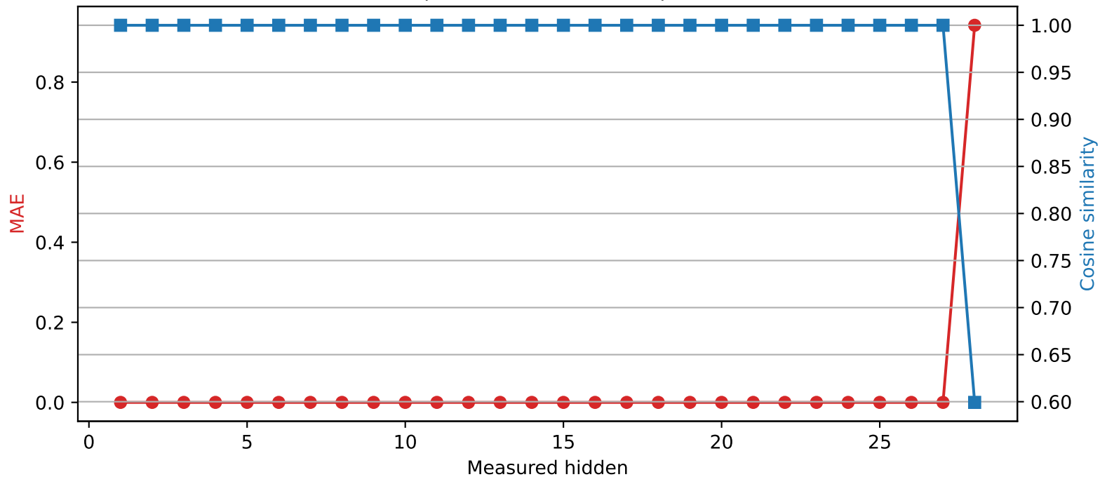
Llama-3.2-3B | Quantized layer 27 | float32 \rightarrow int2
