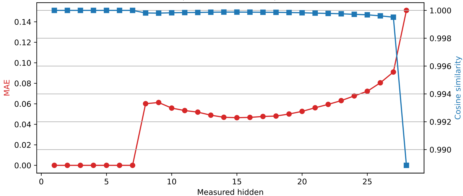
Llama-3.2-3B | Quantized layer 7 | float32 \rightarrow int2
