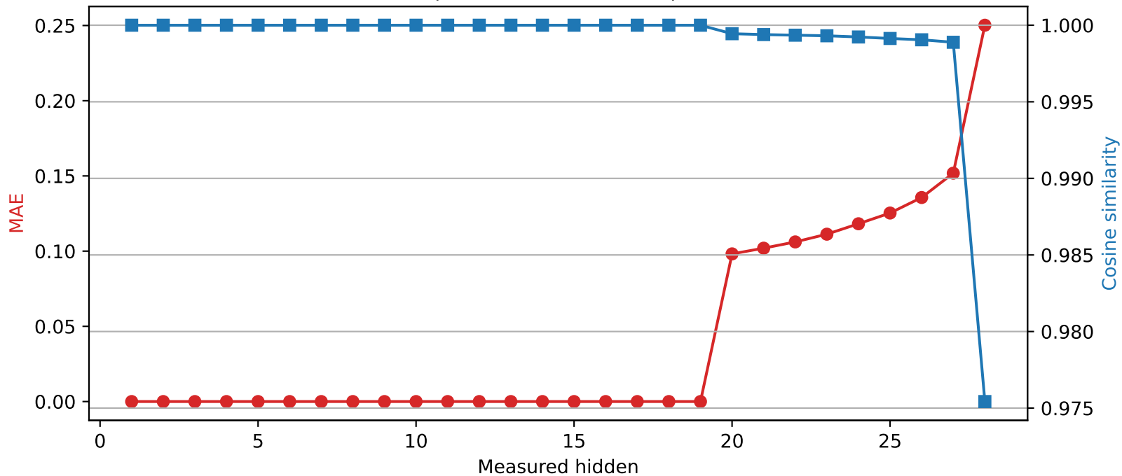
Llama-3.2-3B | Quantized layer 19 | float32 \rightarrow int2
