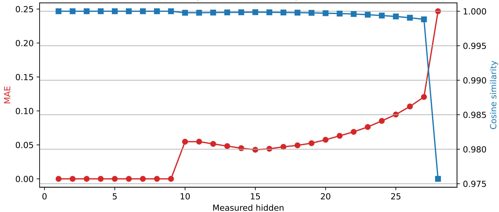
Llama-3.2-3B | Quantized layer 9 | float64 \rightarrow int2
