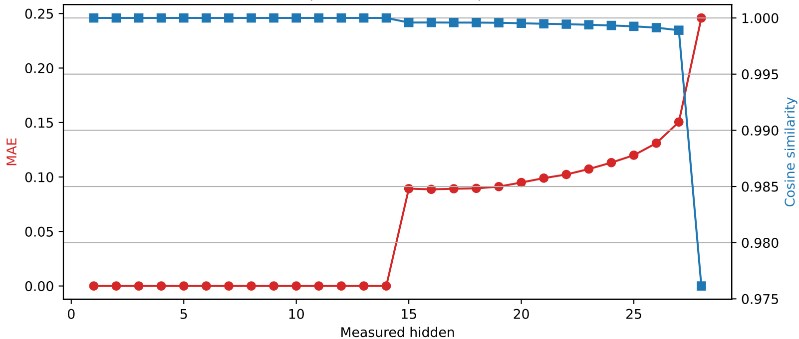
Llama-3.2-3B | Quantized layer 14 | float64 \rightarrow int2
