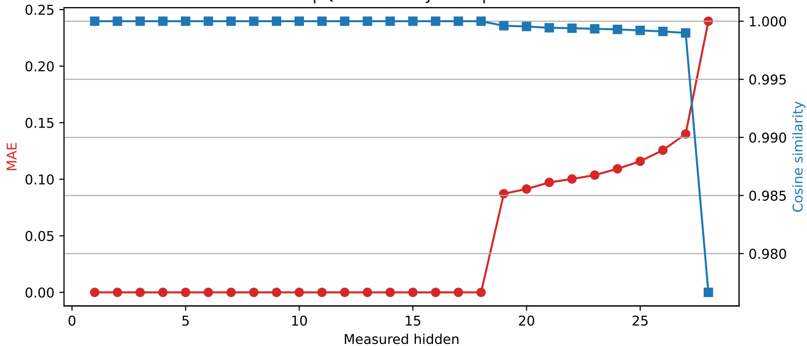
Llama-3.2-3B | Quantized layer 18 | float64 \rightarrow int2
