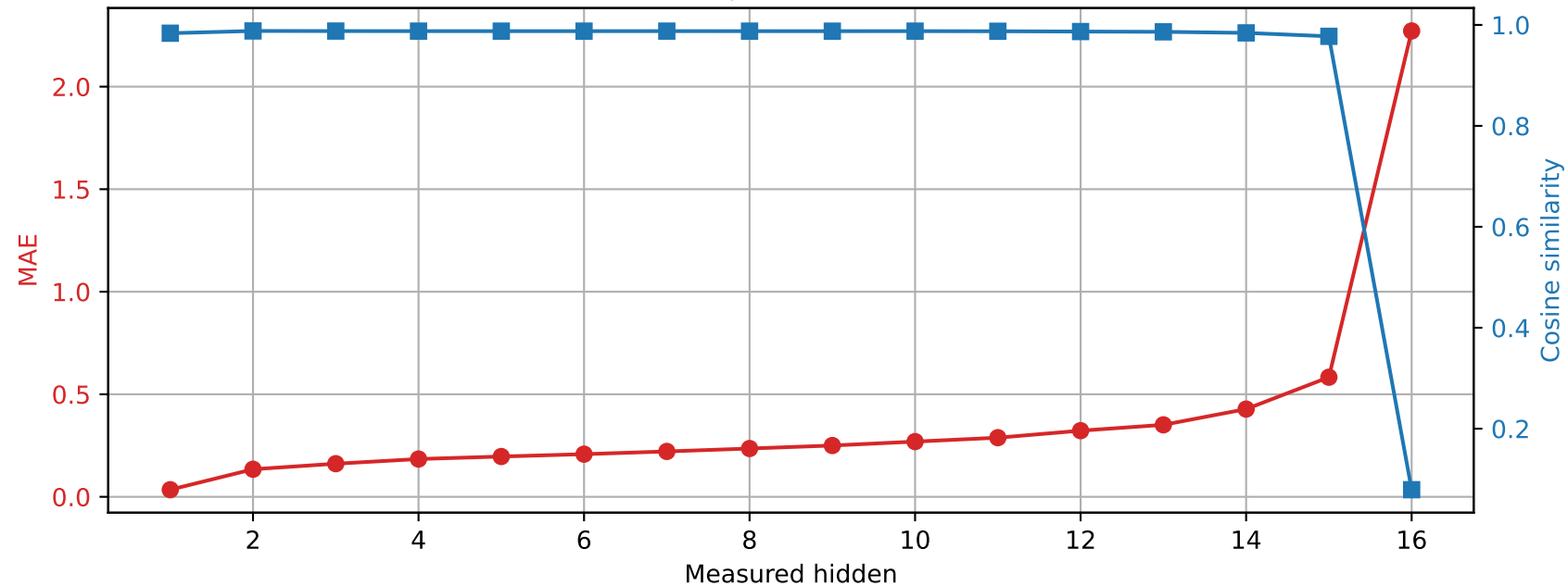
Llama-3.2-1B | Prompt 0 Spared layer 4 | Unquantized vs hybrid
