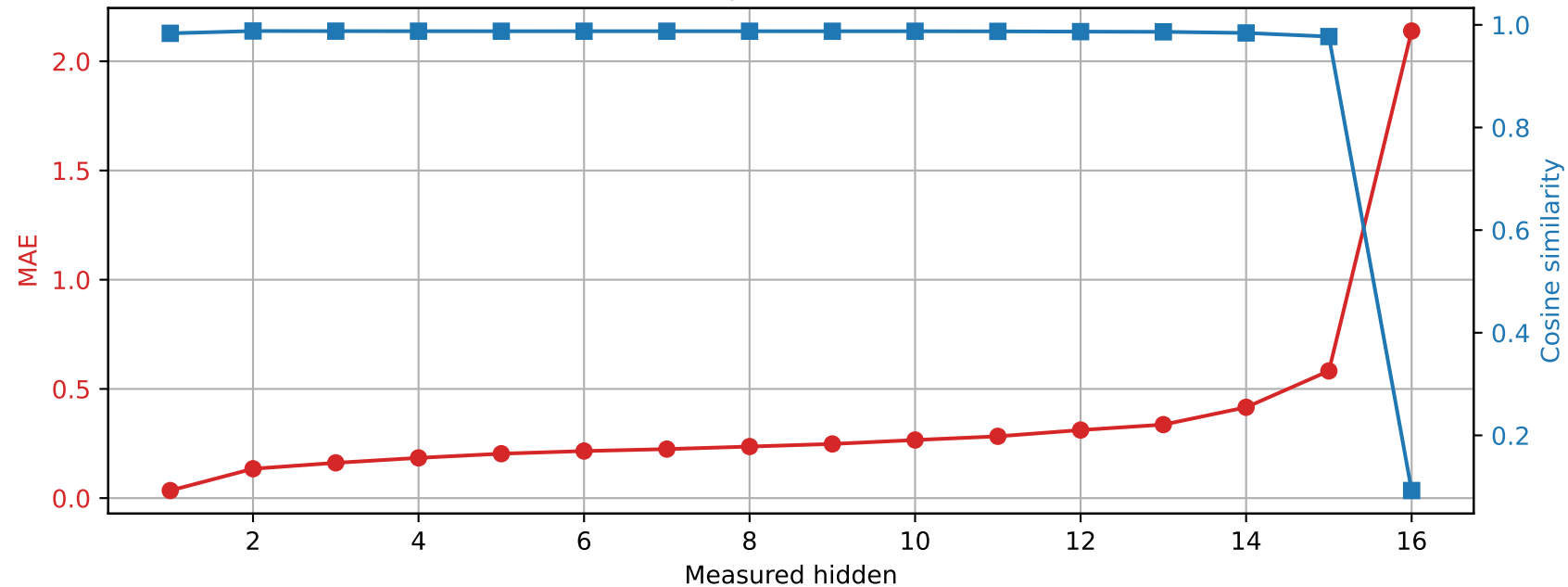
Llama-3.2-1B | Prompt 0 Spared layer 6 | Unquantized vs hybrid
