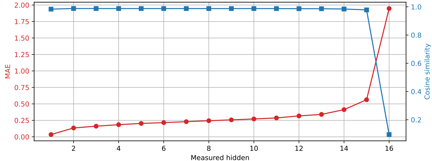
Llama-3.2-1B | Prompt 0 Spared layer 7 | Unquantized vs hybrid
