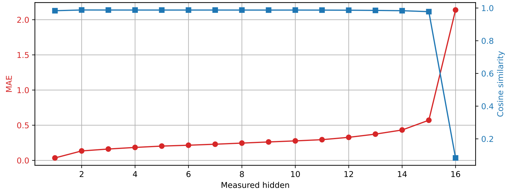
Llama-3.2-1B | Prompt 0 Spared layer 12 | Unquantized vs hybrid
