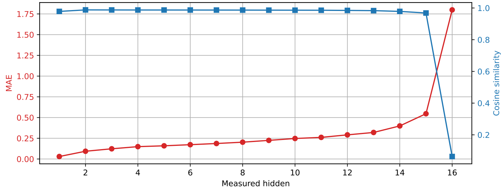
Llama-3.2-1B | Prompt 1 Spared layer 4 | Unquantized vs hybrid
