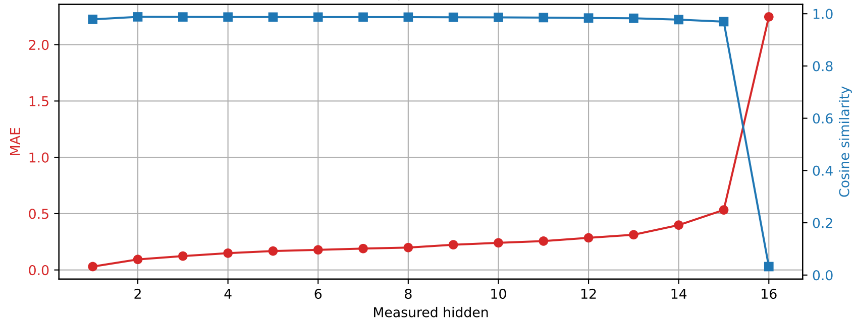
Llama-3.2-1B | Prompt 1 Spared layer 7 | Unquantized vs hybrid
