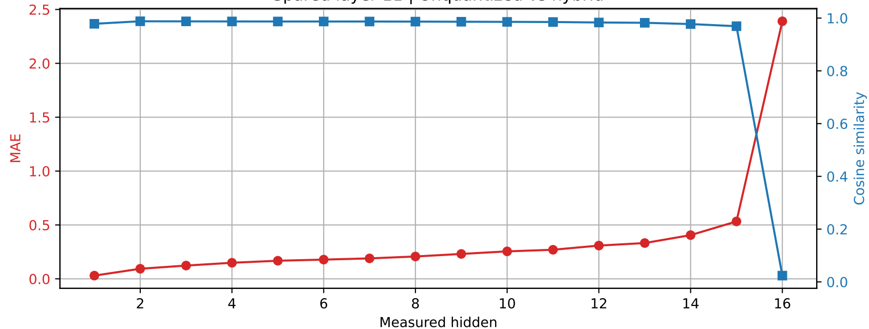
Llama-3.2-1B | Prompt 1 Spared layer 11 | Unquantized vs hybrid
