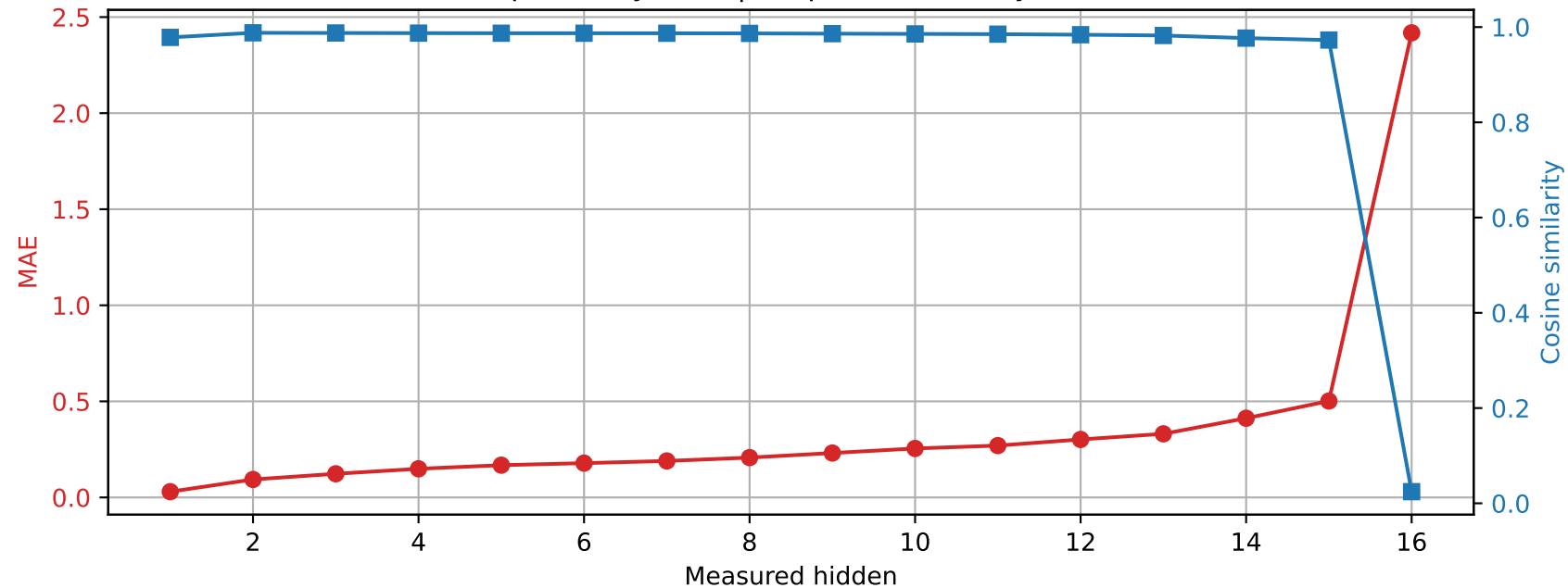
Llama-3.2-1B | Prompt 1 Spared layer 14 | Unquantized vs hybrid
