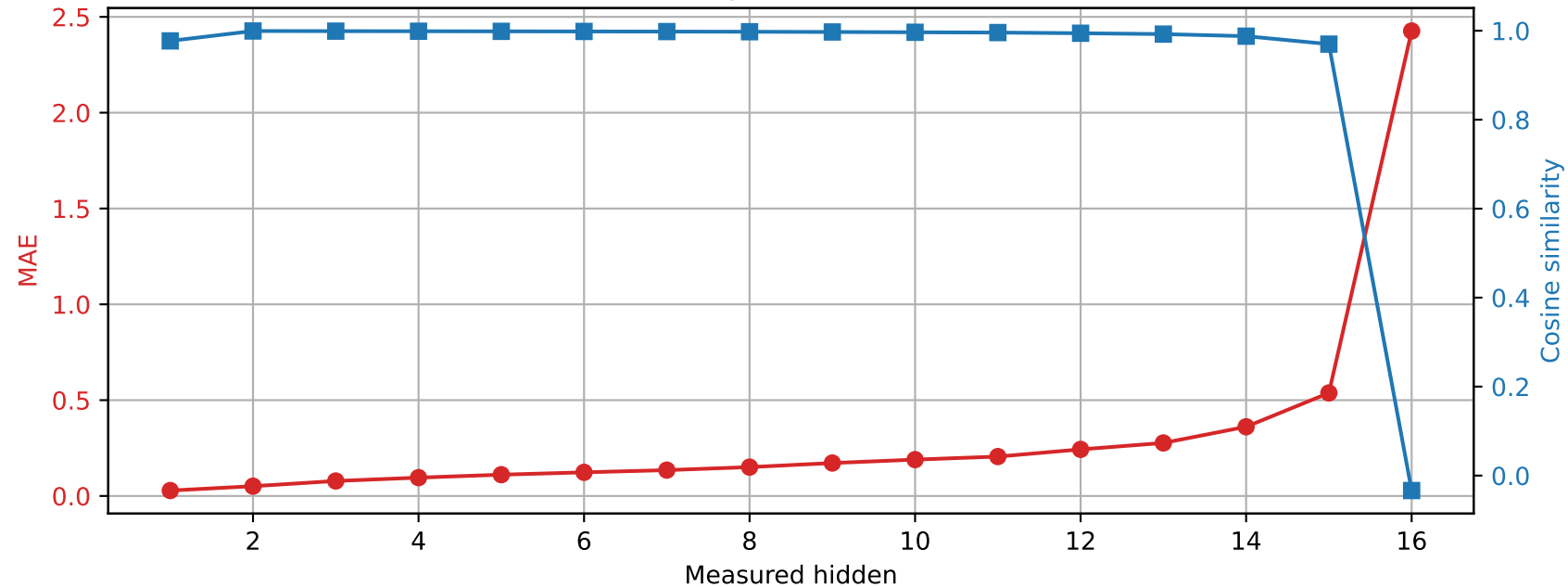
Llama-3.2-1B | Prompt 2 Spared layer 1 | Unquantized vs hybrid
