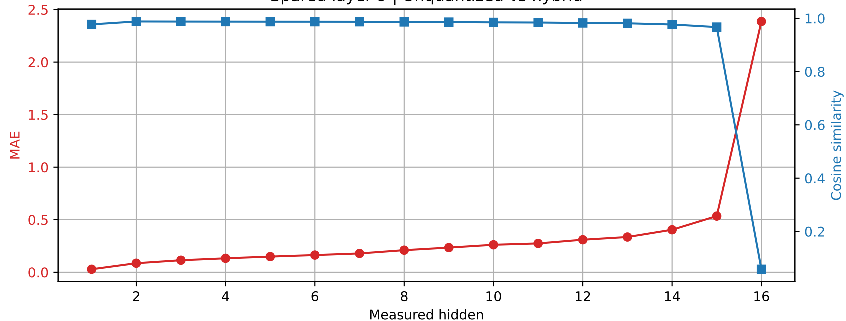
Llama-3.2-1B | Prompt 2 Spared layer 9 | Unquantized vs hybrid
